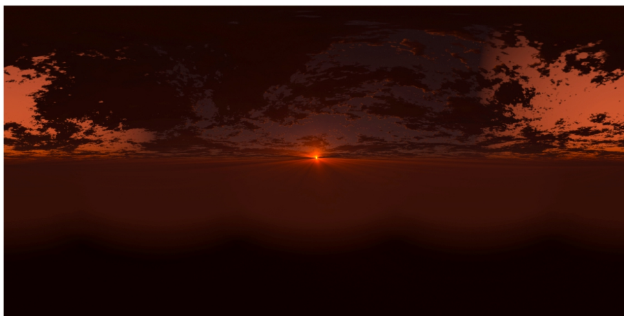
NightSky12
