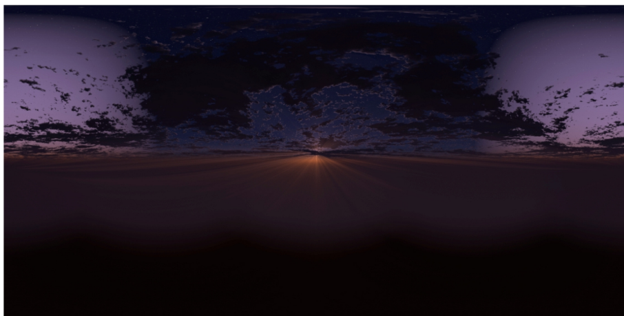
NightSky11
